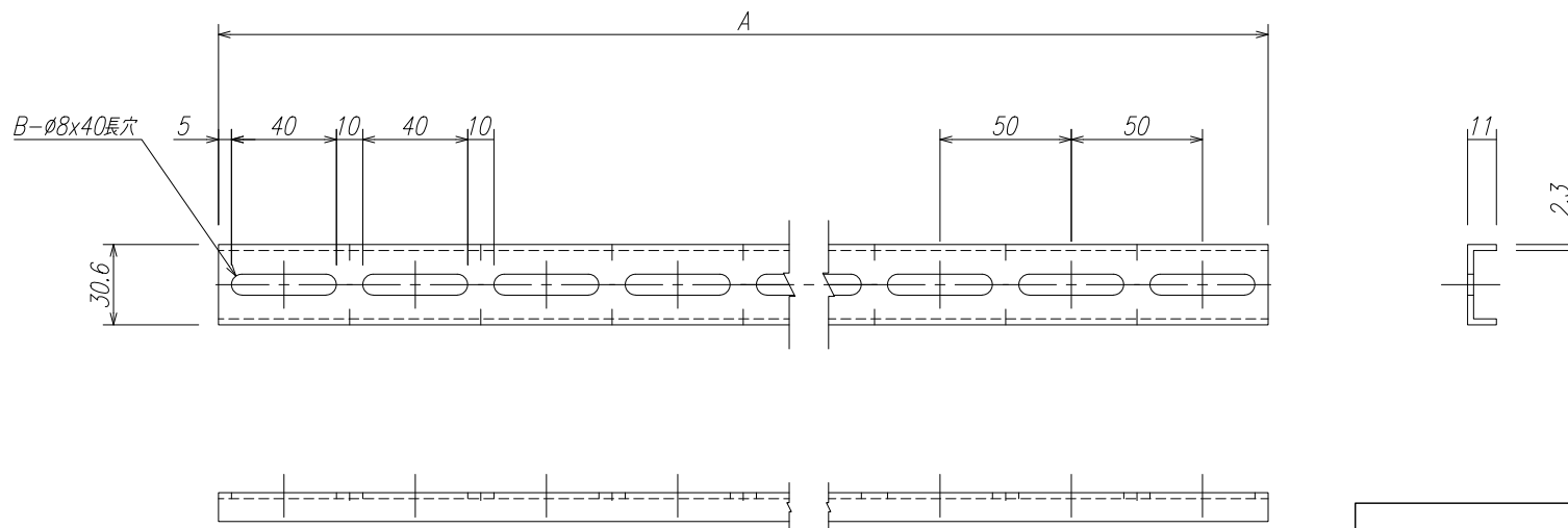
製品仕様図
